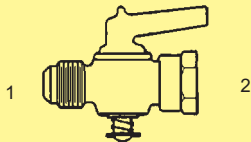
BV-209F - Str. (1) Male 45° Flare (2) Fem. Pipe
