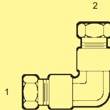
B-IE-85-LB - 90° (1) (2) Tube
