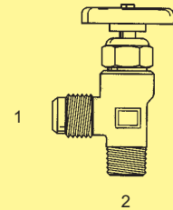
BV-409F - 90° (1) Male 45° Flare (2) Male Pipe
