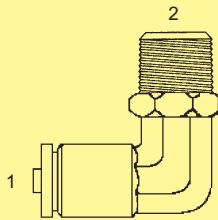
BPC-DOT-2501-S - 90°
