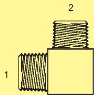
BP-5500 - 90°
