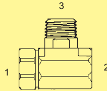
B-POL-2000 - Tee Check
