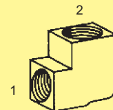
BIF-452 - 90° (1) Fem. Inv. Flare (2) Fem. Pipe
