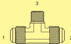
BF-2601-F - Tee
