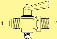
BV-204F - Str. (1) Male 45° Flare (2) Male Pipe
