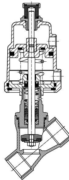
Válvula normalmente abierta
