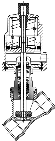
Válvula normalmente cerrada
